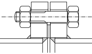
Giunto a flange saldate a sovrapposizione Joint with circular slip-on welded flanges
