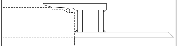
Giunto femmina per tubi C.A.P. Female joint for C.A.P. pipes
